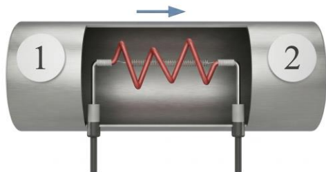
Seção de aquecimento
